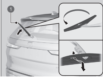
1 Rameno stierača
