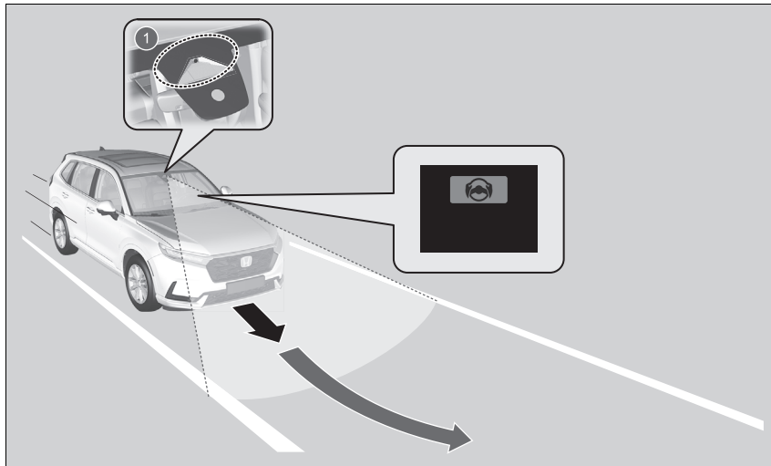
1 Kamera predného snímača: Monitoruje čiary jazdného pruhu
